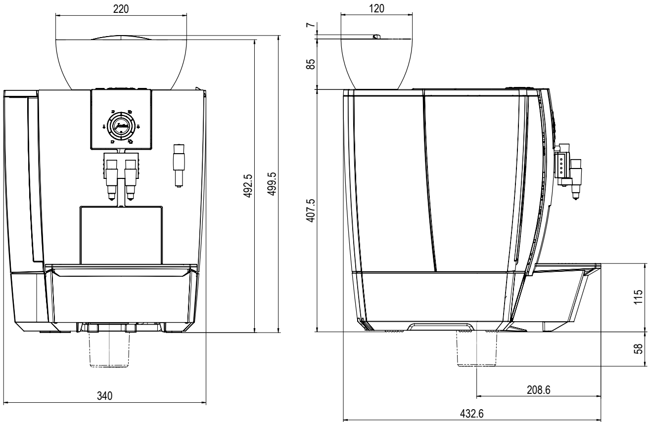
Aufriss
