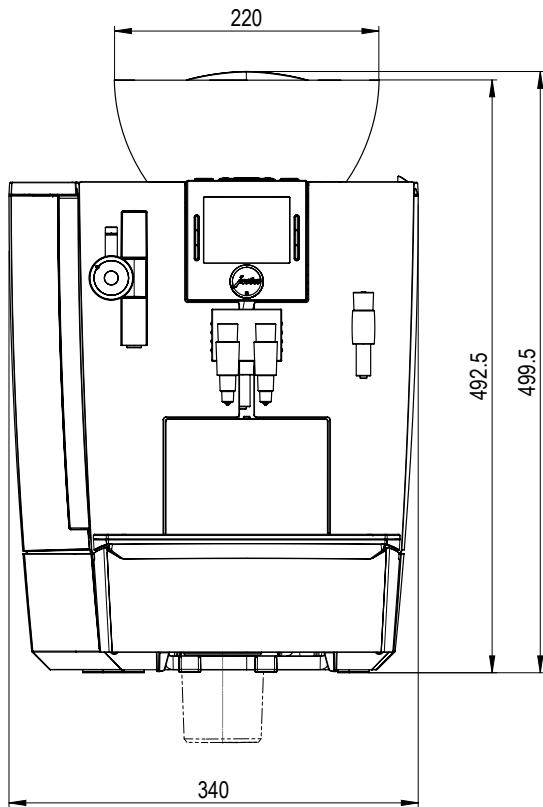
Aufriss
